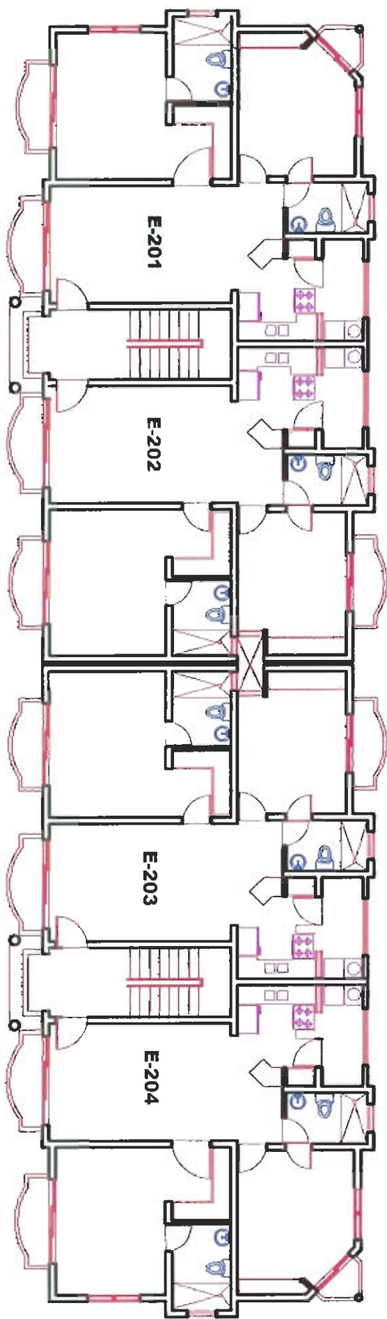
PLANTA ARQ. MODULO - E 2do NIVEL.
