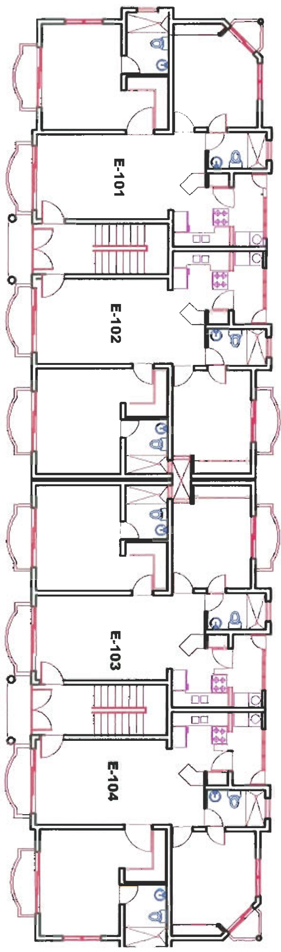
PLANTA ARQ. MODULO - E 1er NIVEL.
